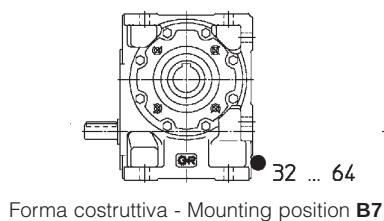
Forma costruttiva - Mounting position B7
