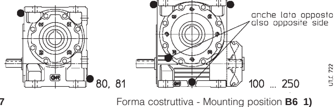
Forma costruttiva - Mounting position B6 1)
