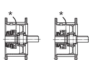
MLA ad attrito friction
